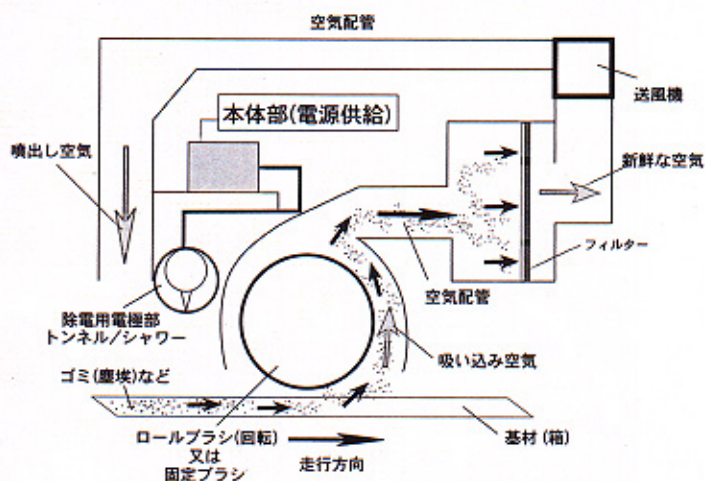
■プラスチック製コンテナやケースなどの除塵装置
